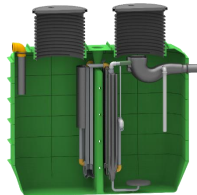
EcoBox SBR 2-20 PE
